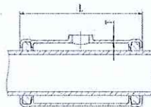
(2) 直管(直身)修补器
