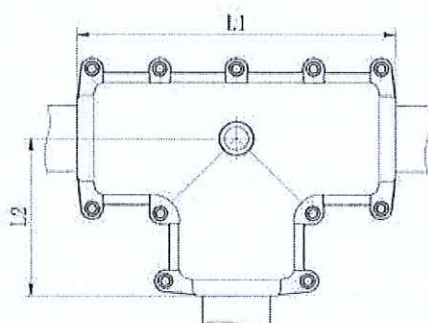
(1) 承插(大头)修补器
