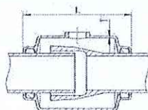
(1) 承插(大头)修补器
