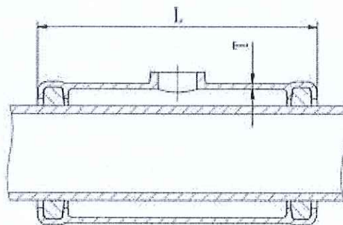
(2) 直管(直身)修补器
